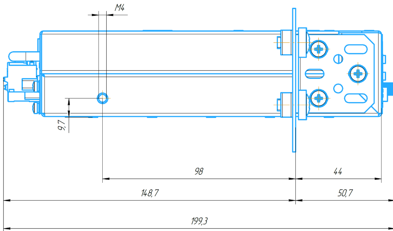
Рисунок Б.4 – Вариант установки устройства с уменьшением монтажной глубины
