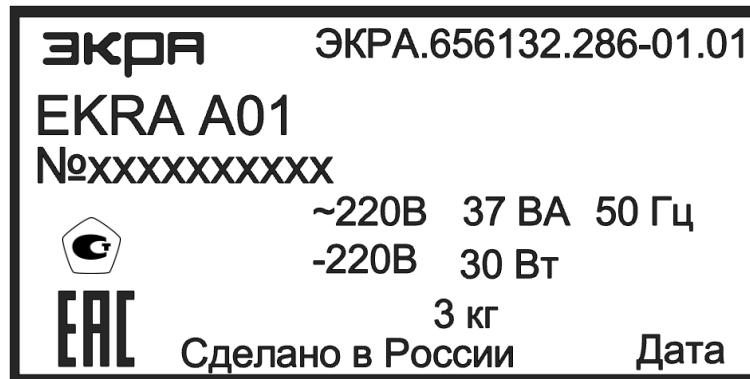
Рисунок 1 – Пример паспортной таблички устройства
