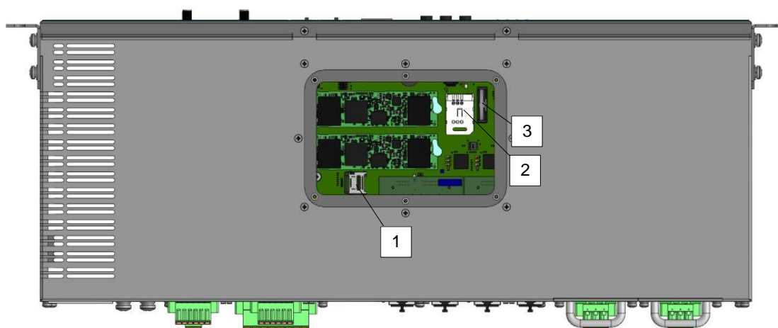
Рисунок 2 – Демонтаж смотровой крышки устройства
