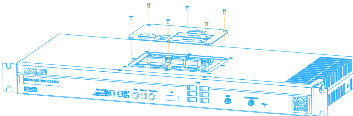
Рисунок 2 – Демонтаж смотровой крышки устройства
