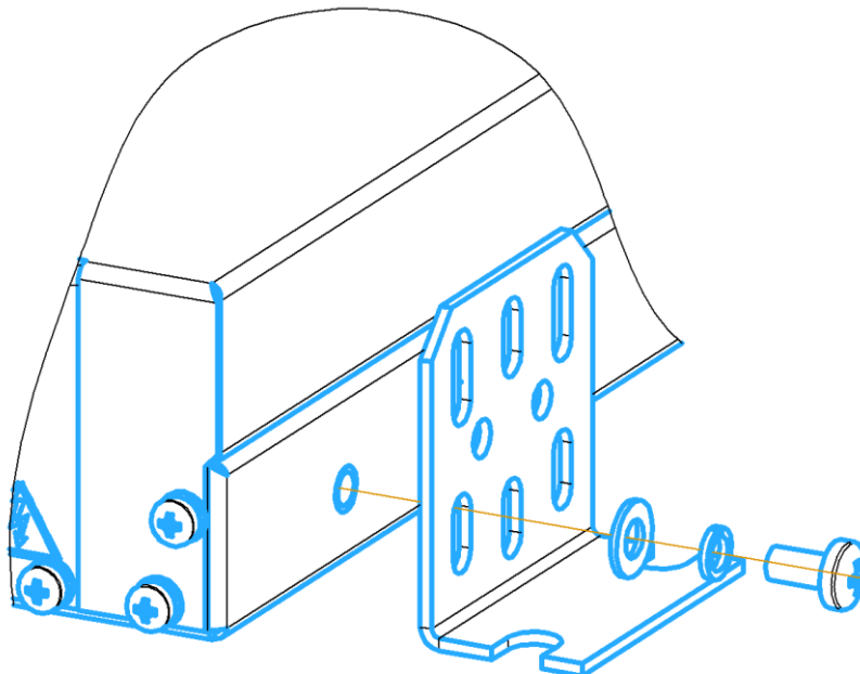
Рисунок 8 – Установка крепежного уголка в задней части устройства
