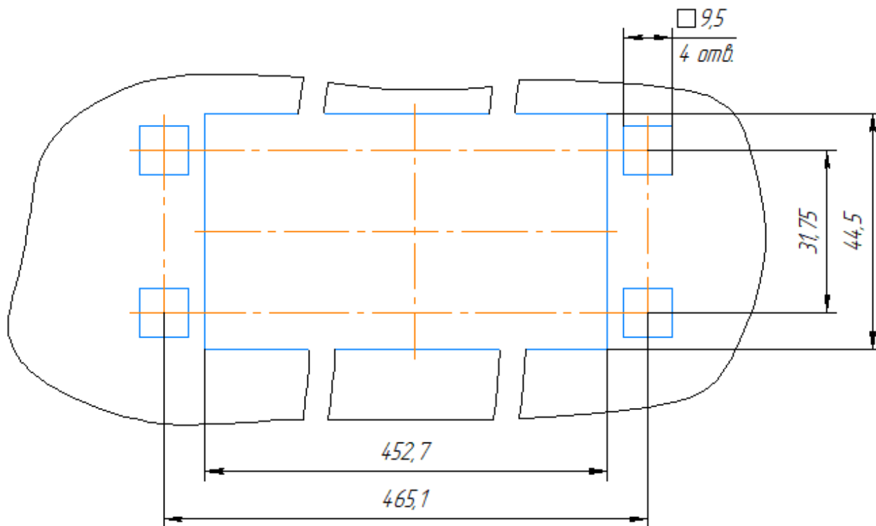
Рисунок Б.1 – Разметка панели под горизонтальный монтаж устройств
