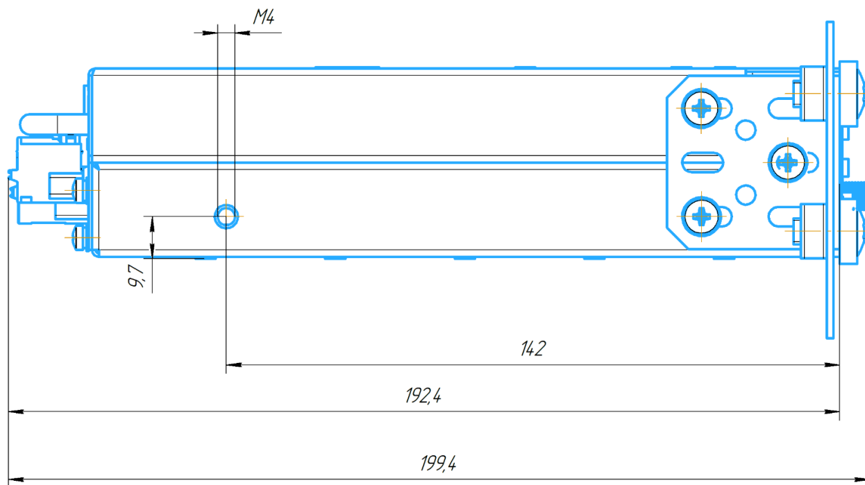
Рисунок Б.3 – Вариант установки устройства на одном уровне с панелью
