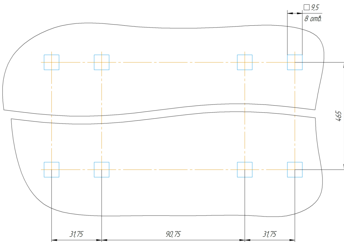
Рисунок Б.2 – Разметка панели под вертикальный монтаж устройства
